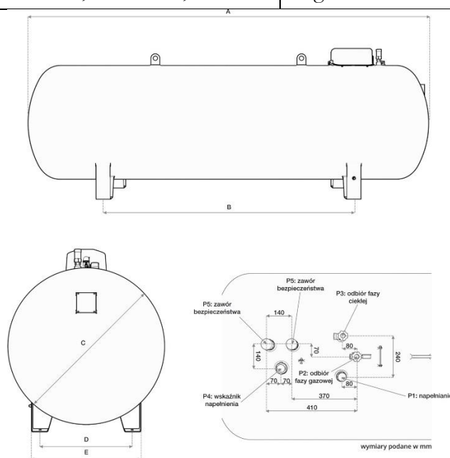
Ryc. 4. Planowane zbiorniki – rysunek techniczny
