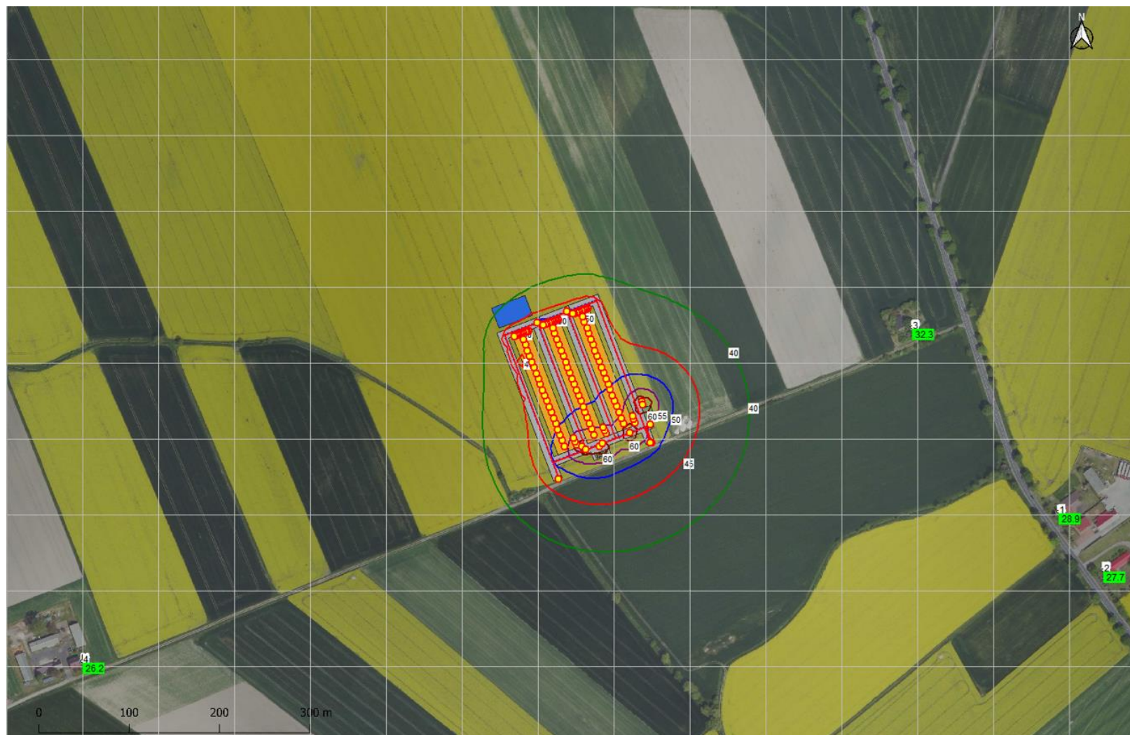
Ryc. 20. Wyniki analizy rozprzestrzeniania hałasu w środowisku w porze dnia – wariant inwestorski
