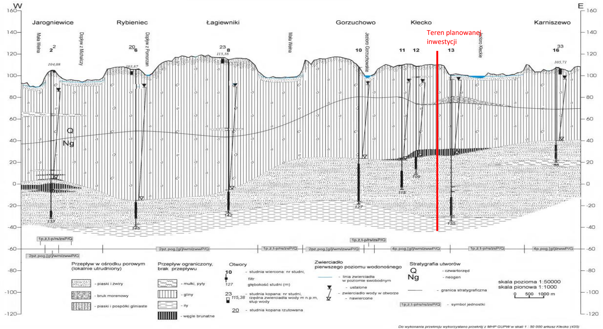
Ryc. 6. Przekrój hydrogeologiczny z zaznaczonym miejscem planowanej inwestycji.
