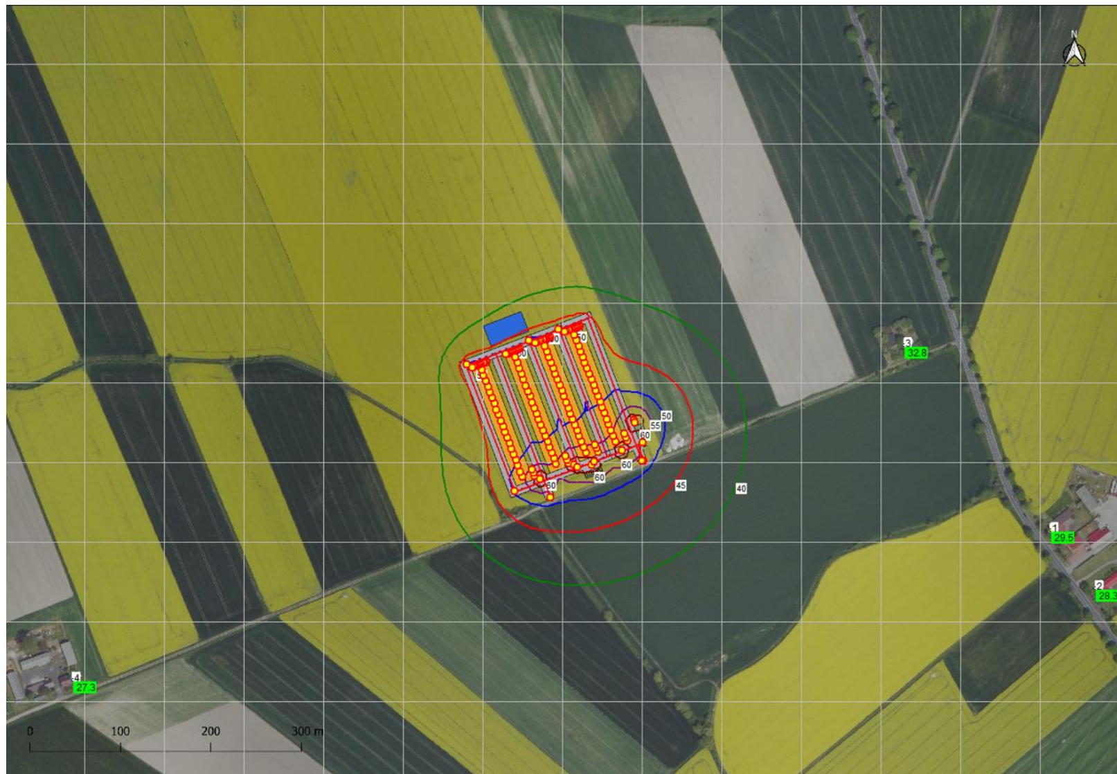
Ryc. 22. Wyniki analizy rozprzestrzeniania hałasu w środowisku w porze dnia – wariant alternatywny
