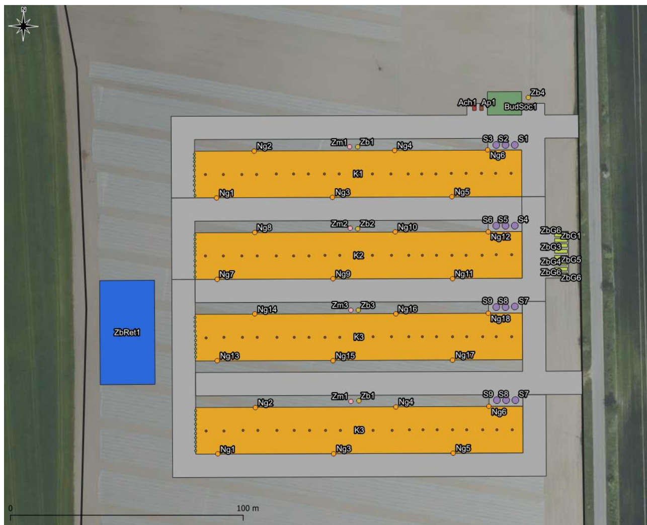
Ryc. 16. Rozmieszczenie obiektów w wariantie alternatywnym
