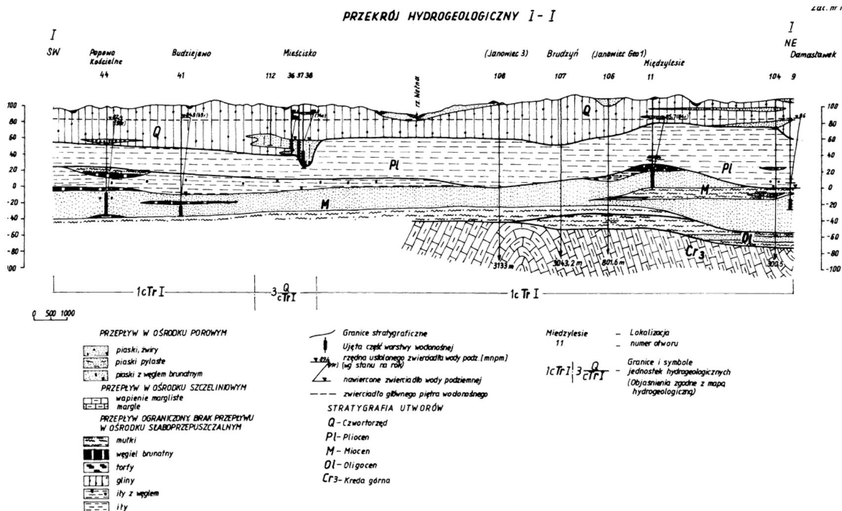
Ryc. 7. Przekrój hydrogeologiczny (planowane przedsięwzięcie zlokalizowane jest na terenie jednostki 1 c Tr I)
