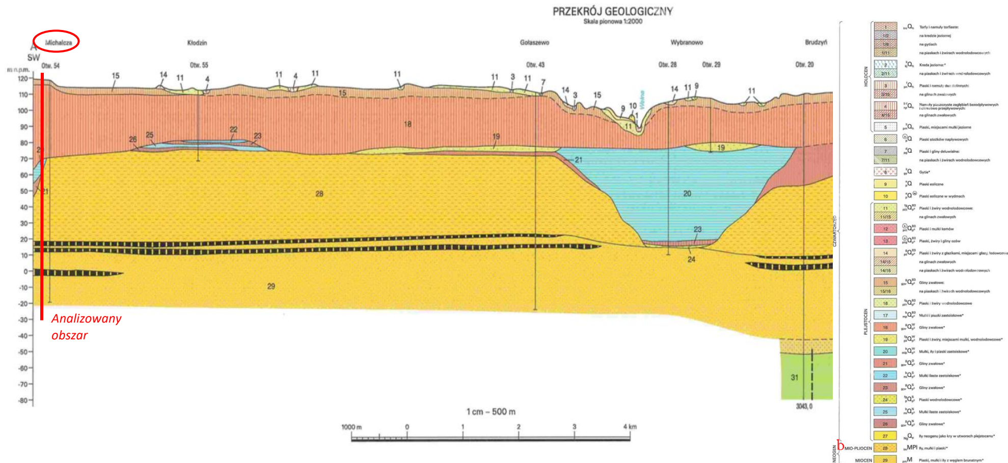
Ryc. 5. Przekrój geologiczny (planowane przedsięwzięcie zlokalizowane jest we wskazanym czerwoną pionową kreską miejscu przekroju)
