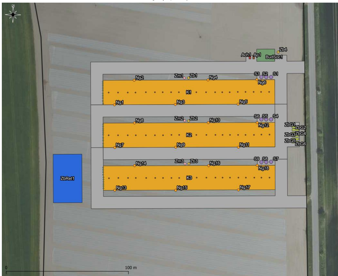
Ryc. 15. Rozmieszczenie obiektów w wariancie inwestorskim
