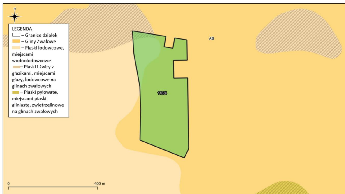
Ryc. 6. Warunki geologiczne rejonu lokalizacji zakładu
