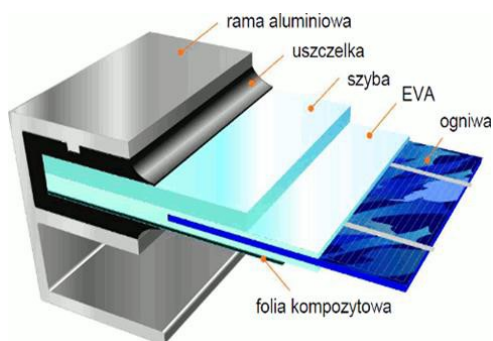
Budowa jednostki wytwórczej farmy fotowoltaicznej
