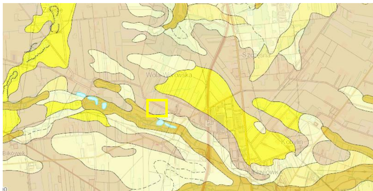
Rysunek 5. Fragment mapy geologicznej 1:50 000 - GRÓJEC (źródło: http://bazagis.pgi.gov.pl )
