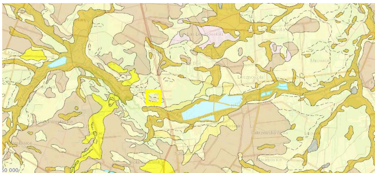
Rysunek 5. Fragment mapy geologicznej 1:50 000 - GRÓJEC (źródło: http://bazagis.pgi.gov.pl )
