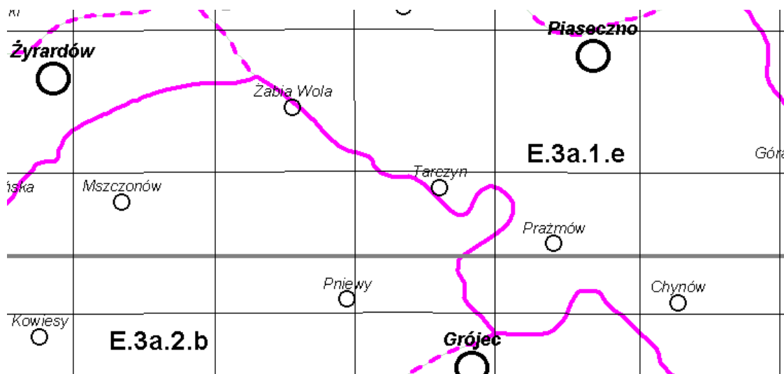
Rysunek 8. Regionalizacja geobotaniczna Polski (źródło: Matuszkiewicz 2008)
