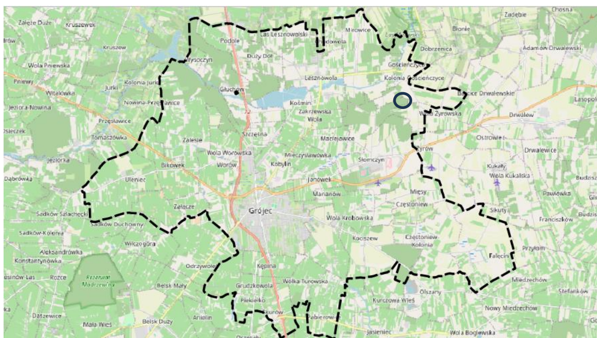
Rysunek 2. Lokalizacja analizowanego obszaru na tle gminy Grójec
