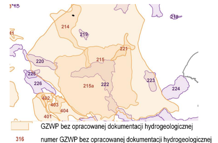
Rysunek 6. Lokalizacja terenu na tle GZWP.
