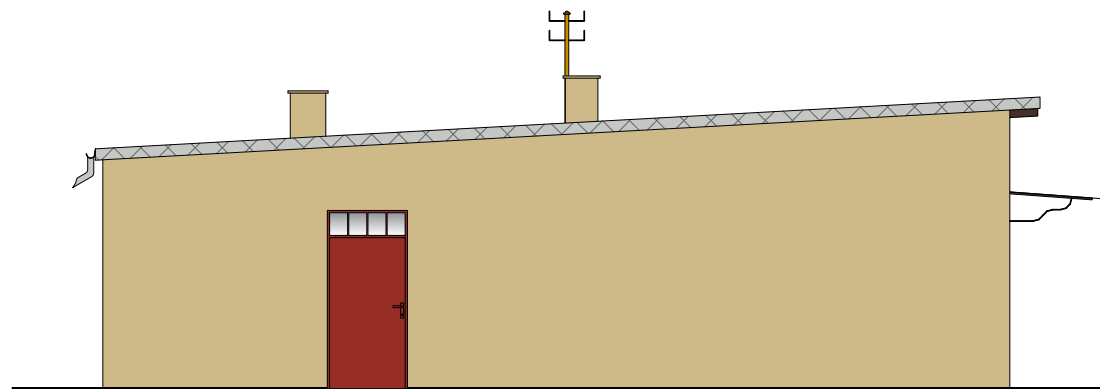
ELEWACJA POŁUDNIOWA
