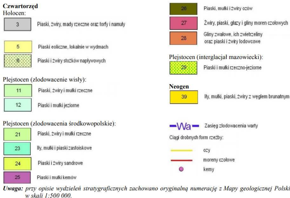
Ryc.11. Mapa geologiczna Polski Arkusz Grójec ( http://bazadata.pgi.gov.pl/data )
