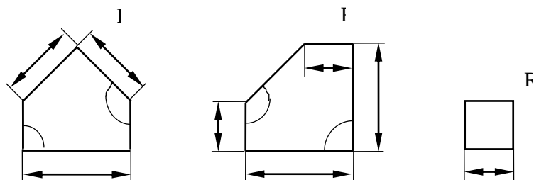
Rysunek 1. Rodzaje płyt chodnikowych betonowych
