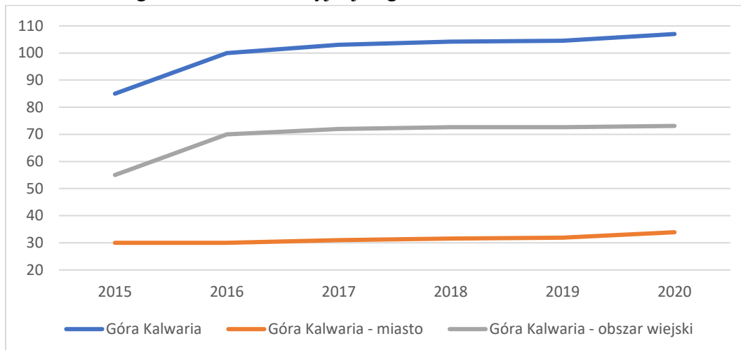
Rysunek 4.5 Długość sieci kanalizacyjnej w gminie Góra Kalwaria w km – lata 2015-2021
