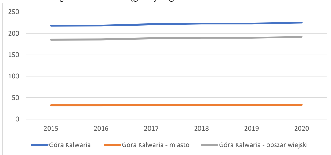
Rysunek 4.1. Długość sieci wodociągowej w gminie Góra Kalwaria w km – lata 2015-2021
