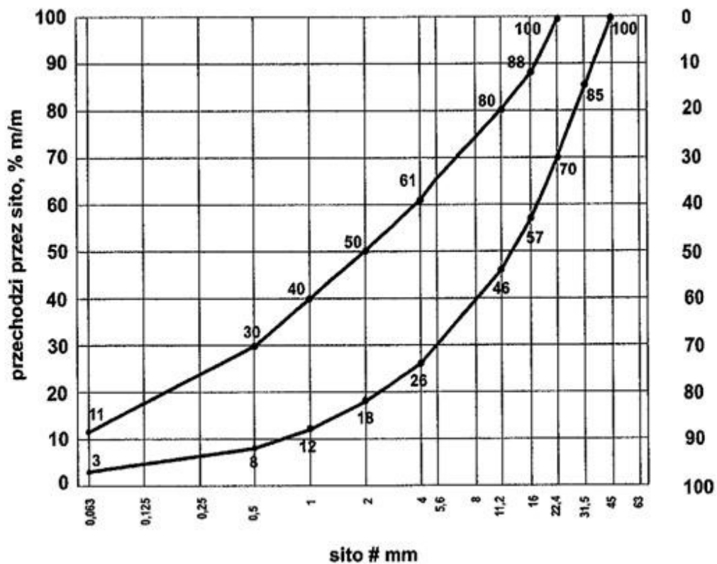
Rys. 1. Krzywe graniczne uziarnienia mieszanki mineralnej 0/31,5 mm
