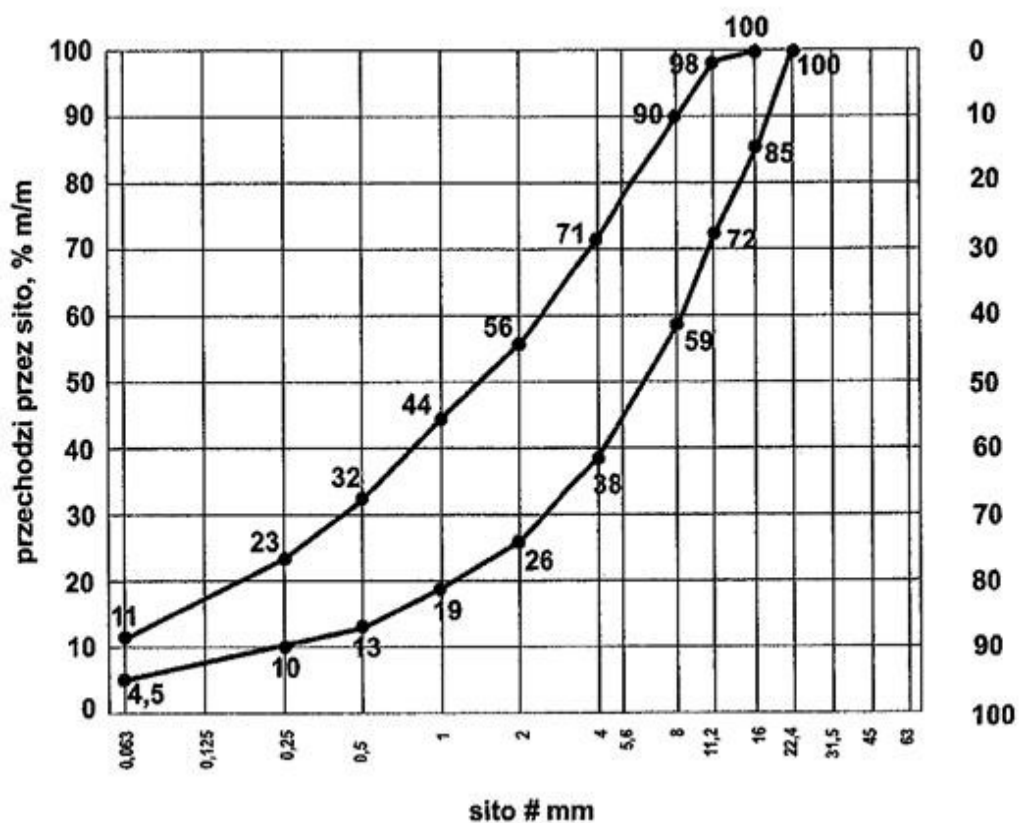
Rys. 3. Krzywe graniczne uziarnienia mieszanki mineralnej 0/16 mm
