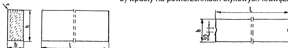
Rys. 1. Wymiarowanie krawężników
