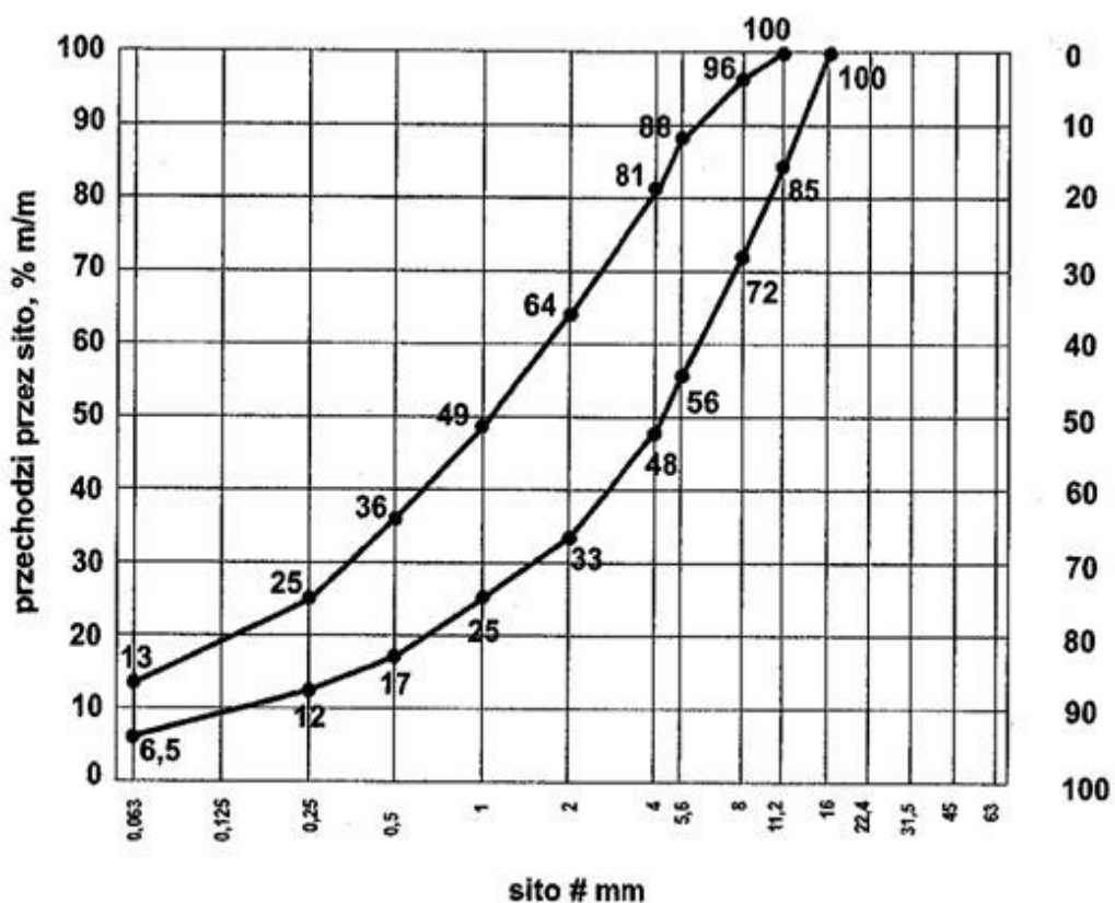
Rys. 4. Krzywe graniczne uziarnienia mieszanki mineralnej 0/11,2 mm
