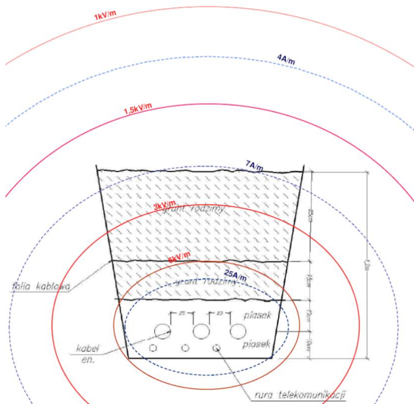
Ryc. 22. Rozkład pola elektromagnetycznego nad przykładową linią kablową (kolorem czerwonym oznaczono izolinie pola elektrycznego, kolorem niebieskim – izolinie pola magnetycznego)
