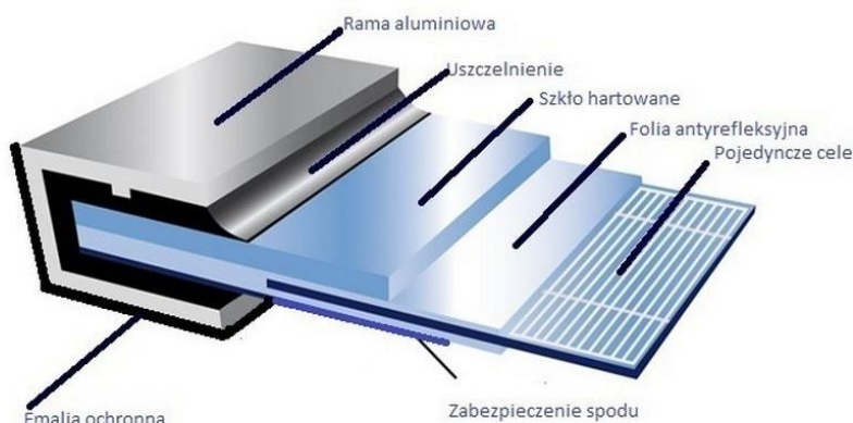
Ryc. 5. Budowa modułu fotowoltaicznego [źródło: www.solwat.pl ]
