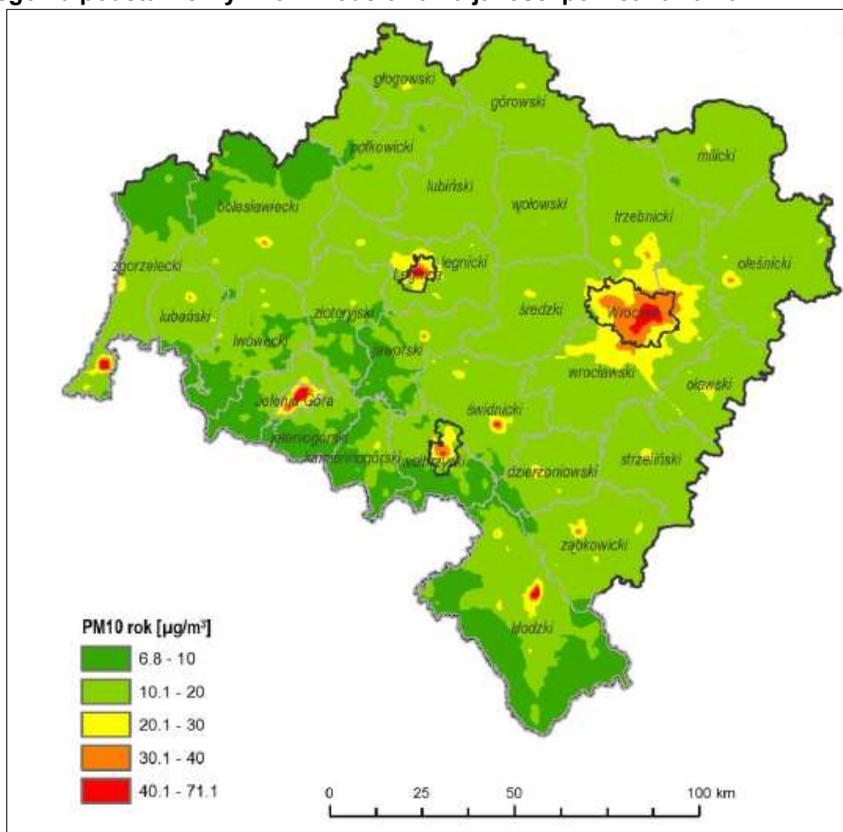
Rysunek 11 Rozkład stężeń średniorocznych pyłu zawieszonego PM 10 na terenie województwa dolnośląskiego na podstawie wyników modelowania jakości powietrza za 2014 r.
