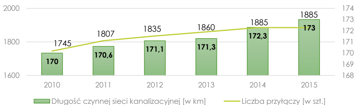
Wykres 14. Długość czynnej sieci kanalizacyjnej [w km] i liczba przyłączy [w szt.] w latach 2010-2015 na terenie gminy Rudna
