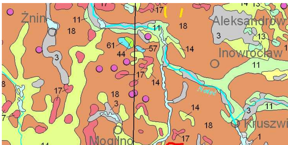
Rys. Fragment mapy geologicznej dla okolic gminy (oryginał w skali 1:500 000)
