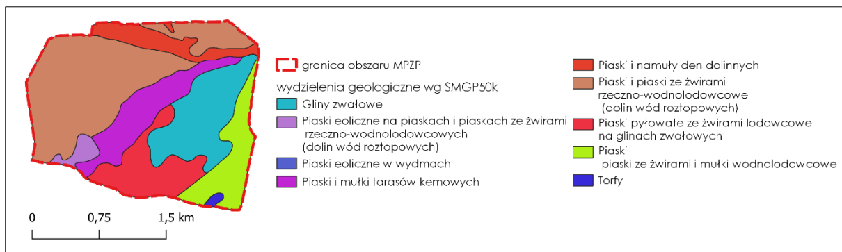
Ryc. 7 Obszar MPZP (obwód Kępa) na tle wydziałów geologicznych wg szczegółowej mapy geologicznej Polski 1:50 000
