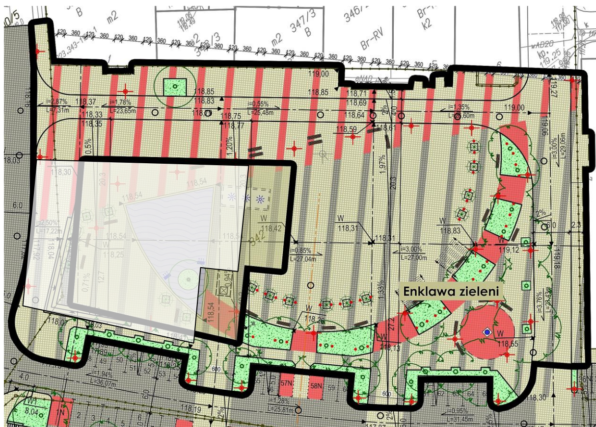
Wrys z dokumentacji (planowany zakres przebudowy)
