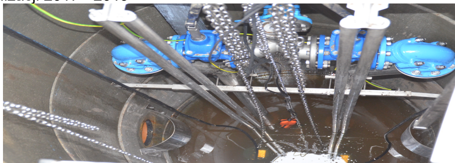
Fotografia nr 30 Sieć kanalizacji sanitarnej wraz z przepompownią w miejscowości Jagodziniec
