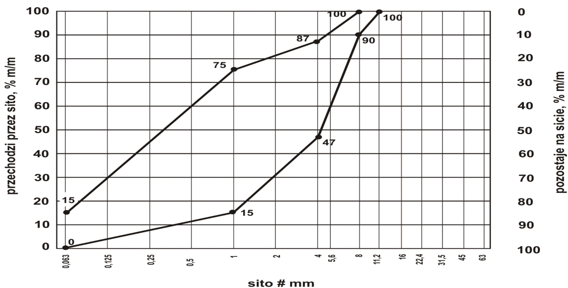
Rys. 1. Uziarnienie mieszanki niezwiązanej 0/8 dla warstwy ulepszonego podłoża
