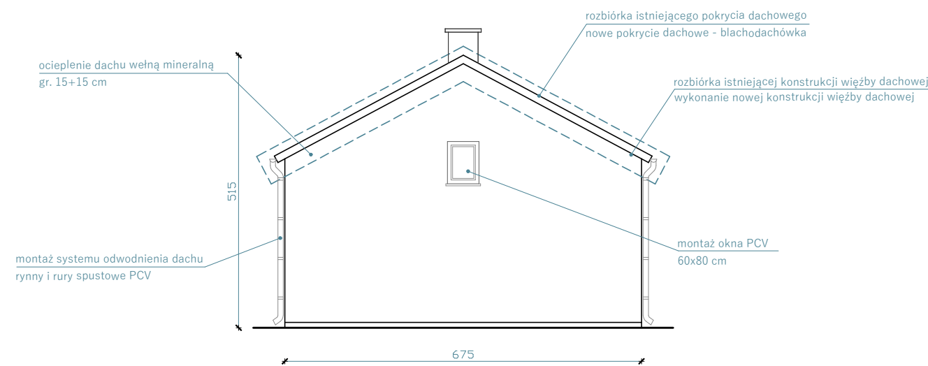
ELEWACJA PÓŁNOCNO-WSCHODNIA
