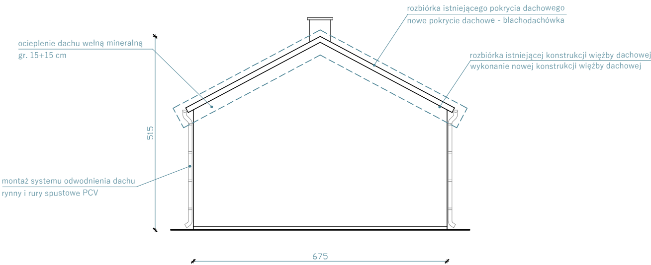
ELEWACJA POŁUDNIOWO-ZACHODNIA
