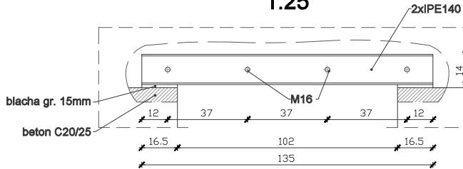
Nadproże N-3 1:25
