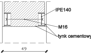
Przekrój A-A 1:25
