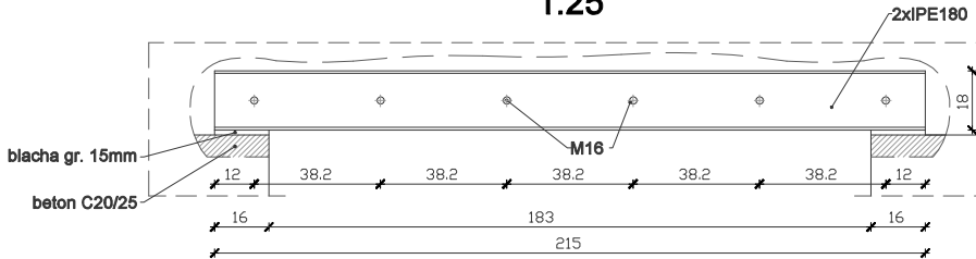
Nadproże N-4 1:25
