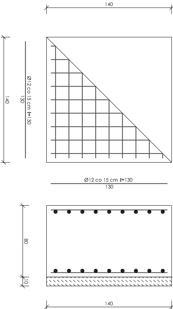
SF2 - Stopa fundamentowa 140 x 140 cm
