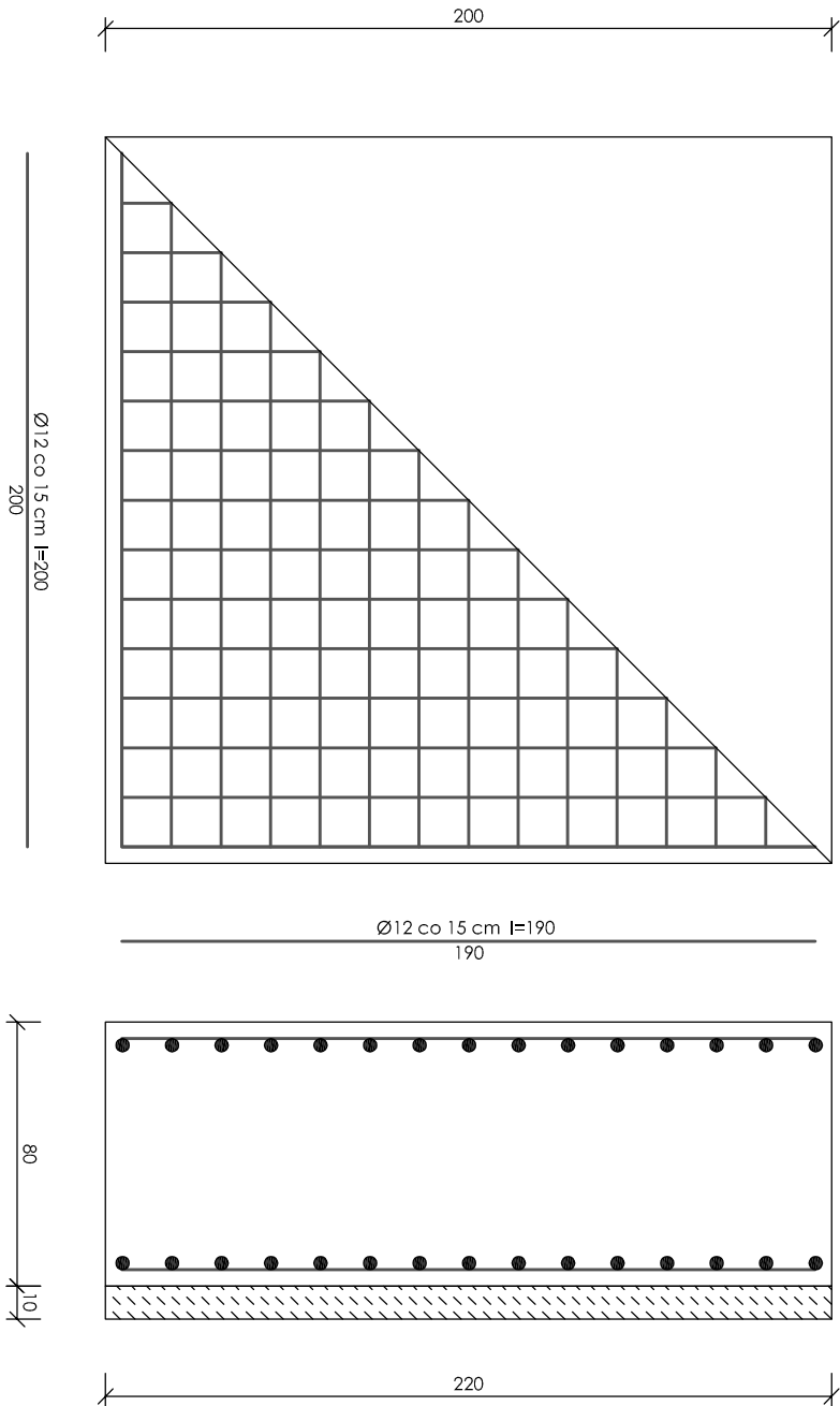
SF1 - Stopa fundamentowa 210 x 200 cm
