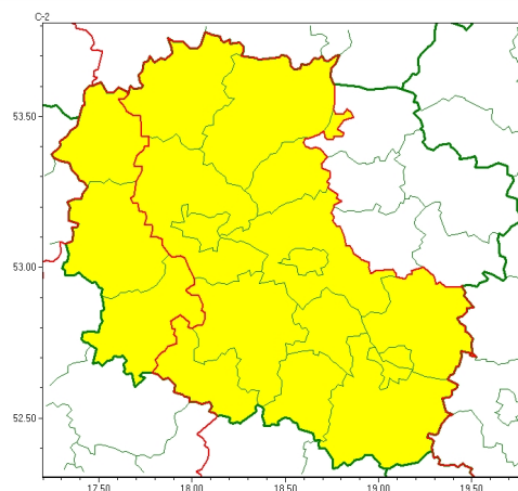
Opady marznące 2025-12-29 06:04
