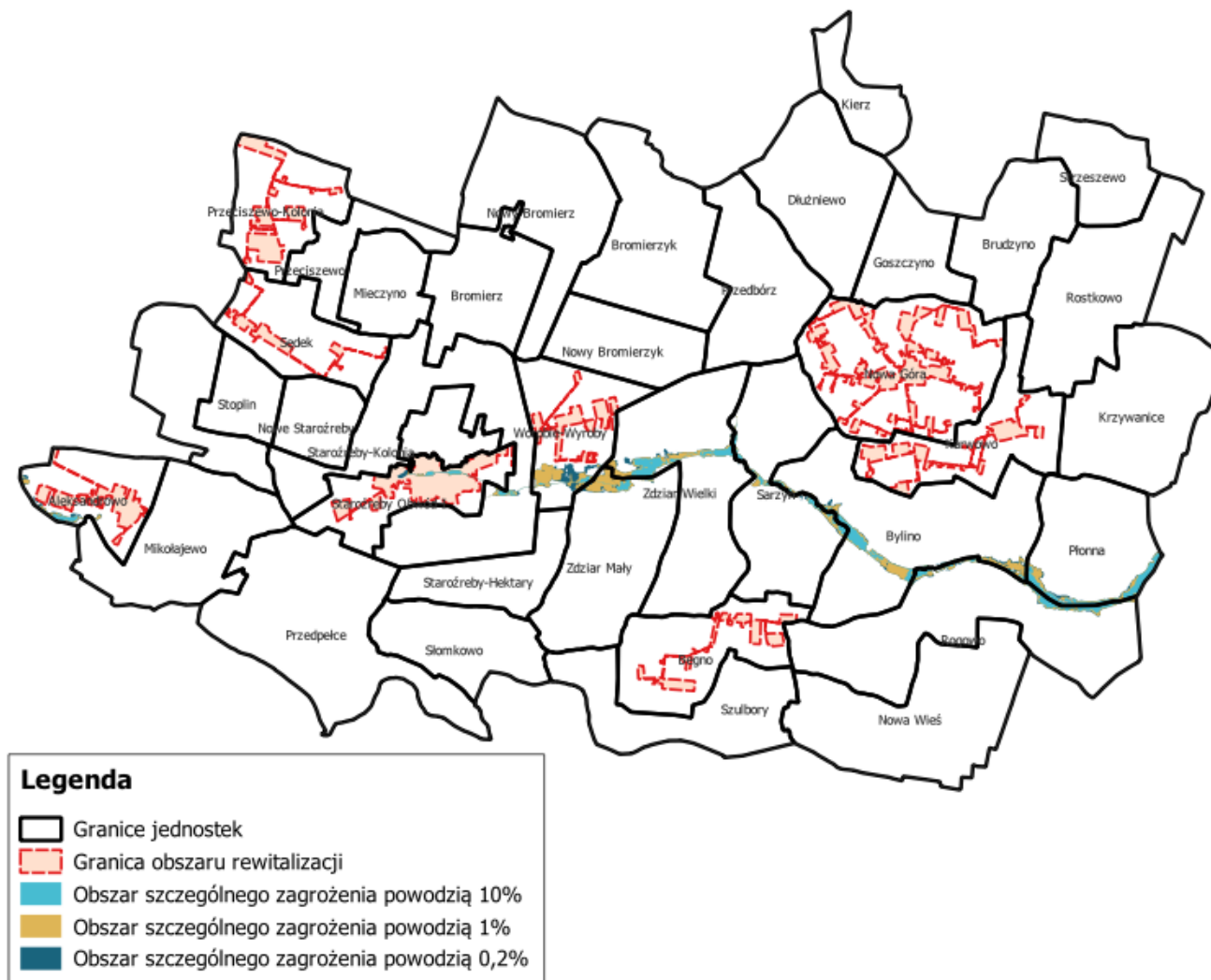
Rysunek 2. Obszary szczególnego zagrożenia powodzią na terenie gminy Staroźreby
