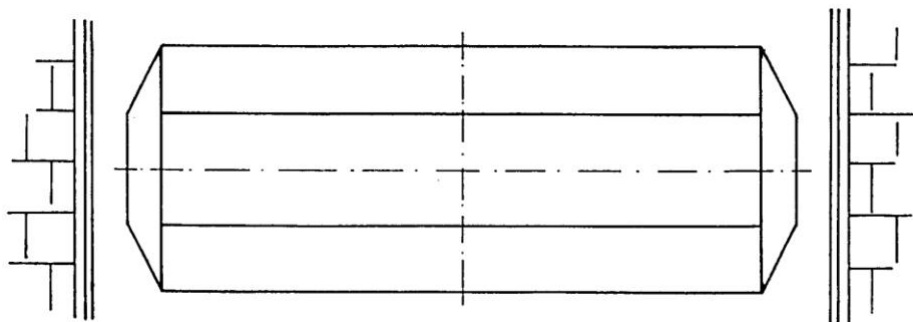
Rys. 2. Przekroje podłużne liniowych progów zwalniających o ograniczonej prędkości przejazdu 25 \div 30 km/h (wg [23])
