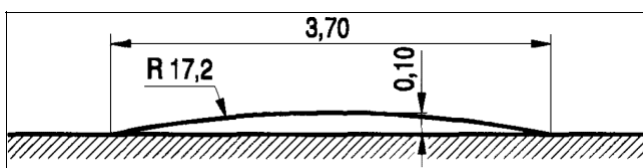
Rys. 2. Przekroje podłużne liniowych progów zwalniających o ograniczonej prędkości przejazdu 25 \div 30 km/h (wg [23])
