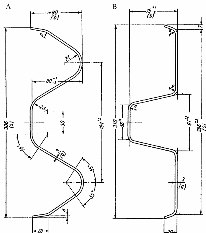
stalowych typu A i B
