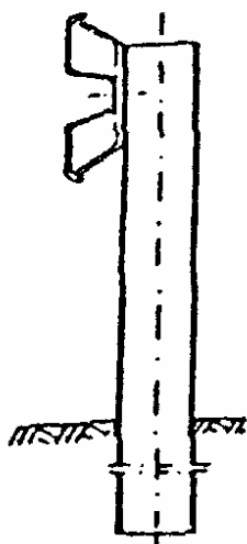
a) bezprzekładkowa wysięgnikowa
