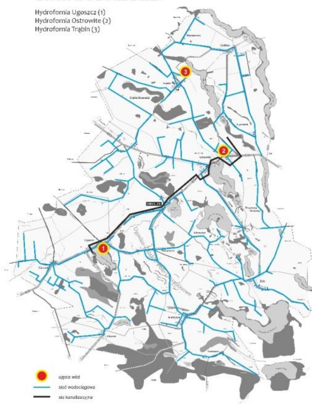
Rys. 31. Schemat sieci wodociągowej w gminie Brzuze
