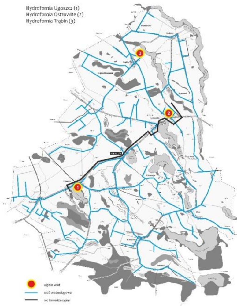
Rys.31. Schemat sieci wodociągowej w gminie Brzuze
