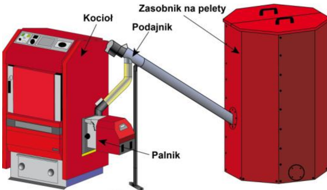
Rysunek 10 Schemat kotła na biomasę
