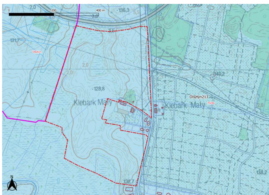
Ryc.11. Położenie obszaru opracowania na tle granic GZWP 213 Olsztyn.
