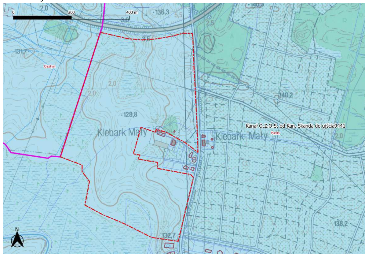
Ryc.6. Położenie obszaru opracowania na tle zlewni elementarnych.
