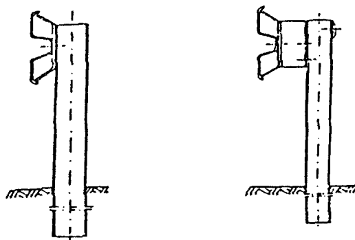
Załącznik 11.2 Bariery ochronne stalowe skrajne z prowadnicą z profilowanej taśmy stalowej stosowane na odcinkach dróg,
