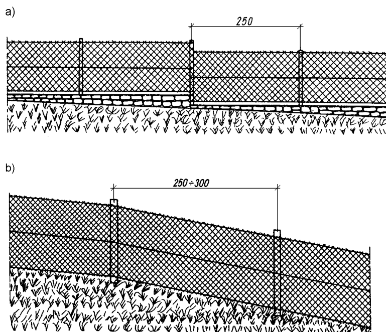
Rys. 6. Przykład ustawienia ogrodzenia siatkowego na terenie pochyłym (wg [6]) Ogrodzenie ze stopniami wysokości 25÷30 cm (przy spadku terenu od 1:16 do 1:30) Ogrodzenie równoległe do terenu
