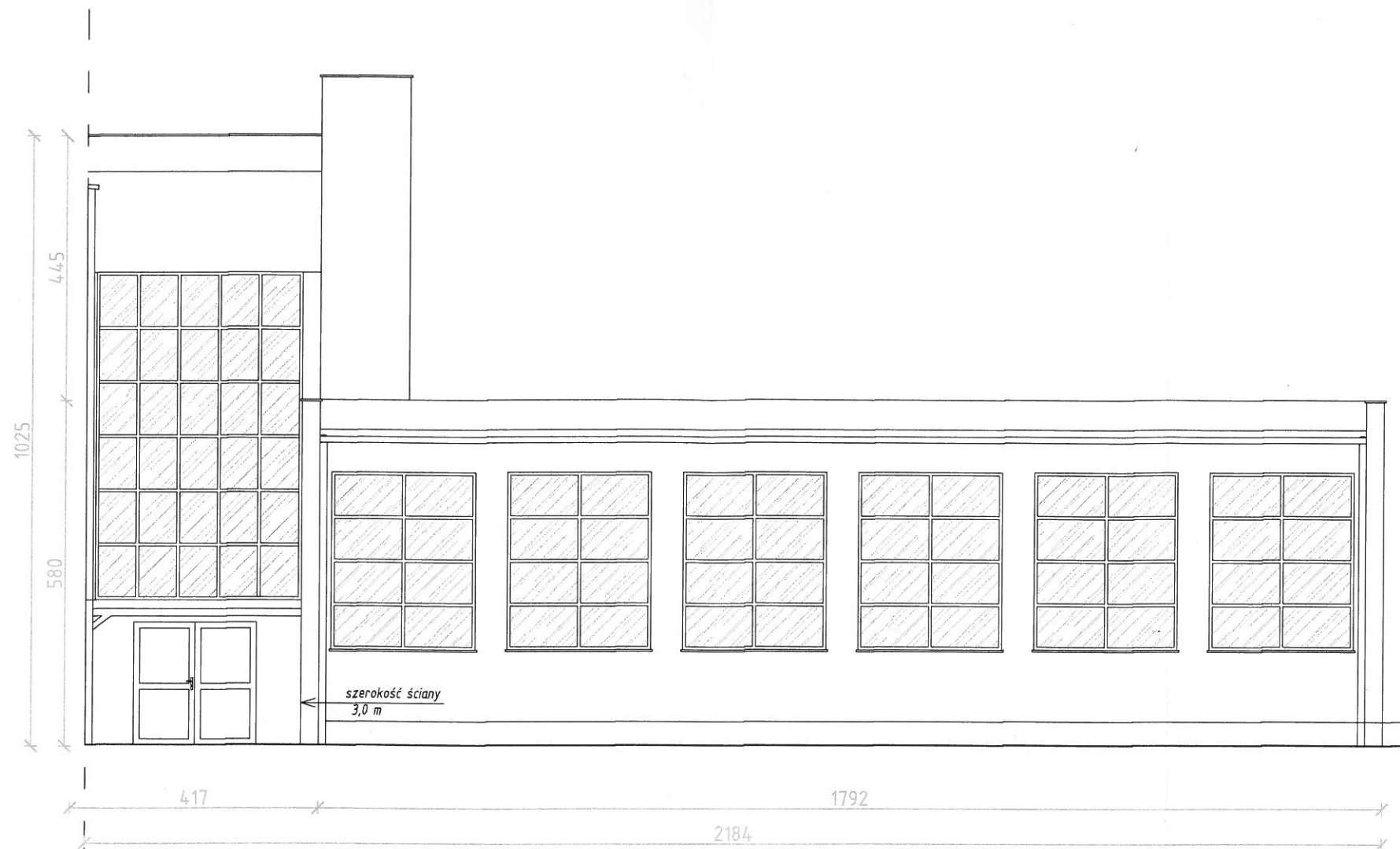
ELEWACJA E
