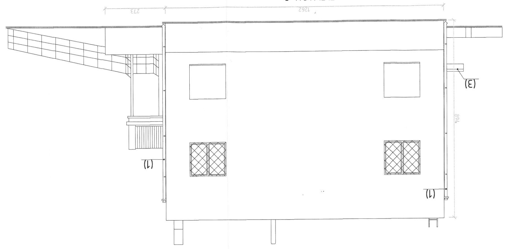
ELEWACJA C
