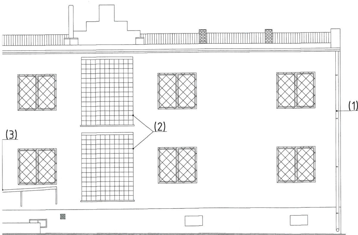
ELEWACJA D
