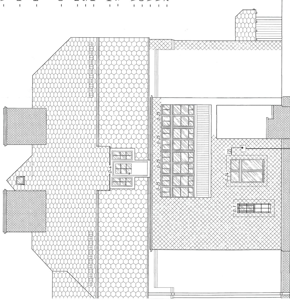
ELEWACJA ZACHODNIA
