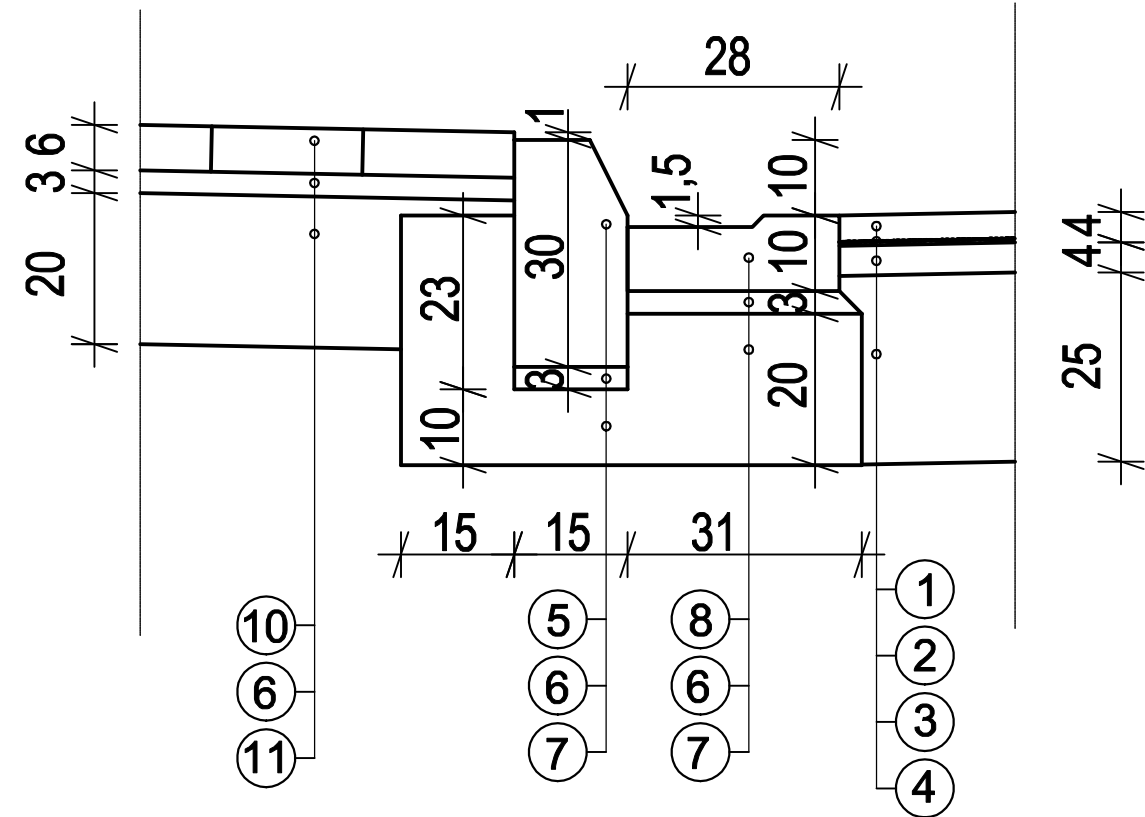
Szczegół połączenia jezdni i chodnika
