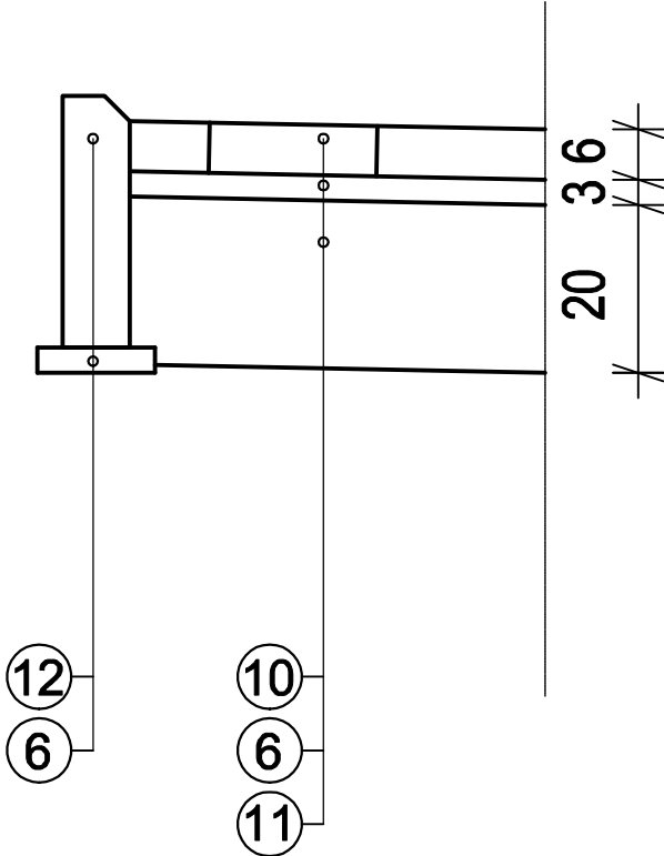
Szczegół chodnika
