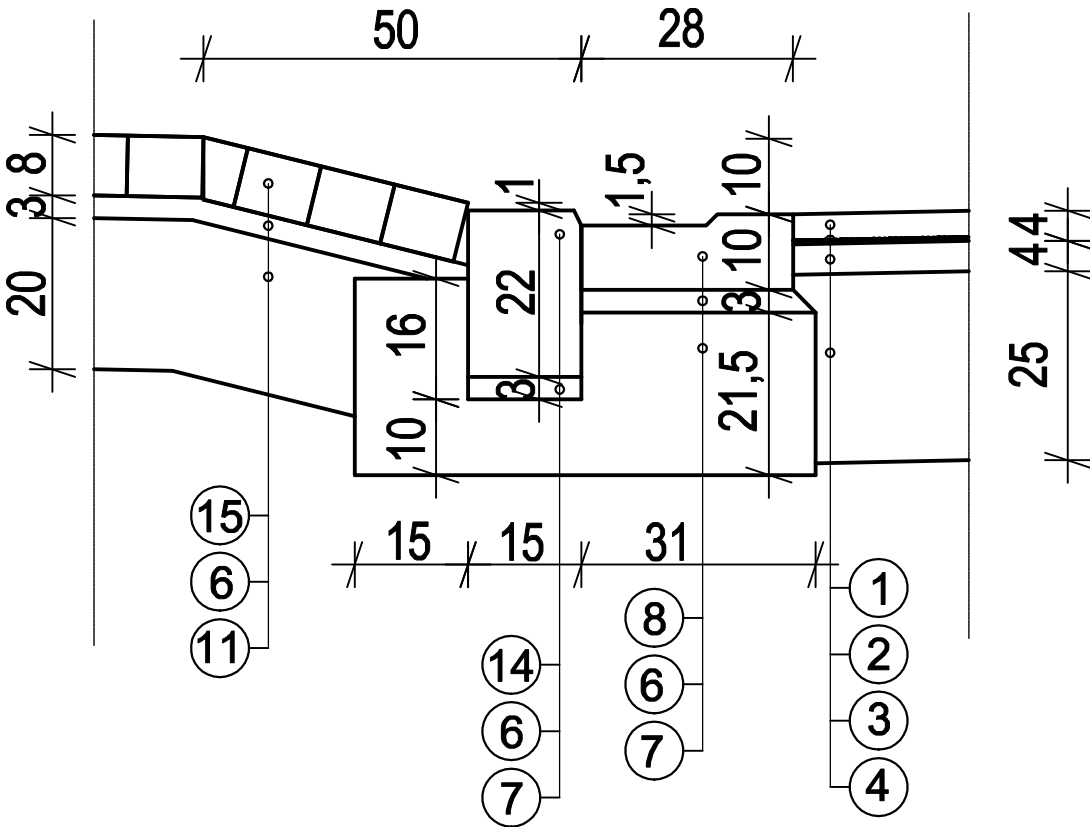
Szczegół zjazdu indywidualnego w chodniku
