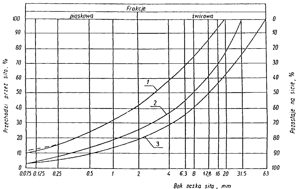
Rysunek 1. dobry uziarnienia kruszyw
