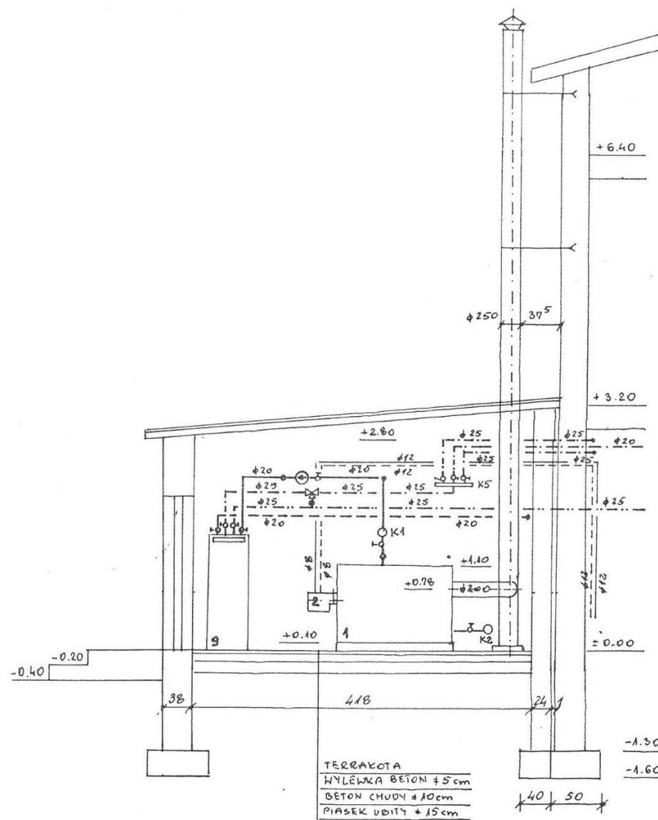
Rys. 3 Poglądowy przekrój istniejącej kotłowni
