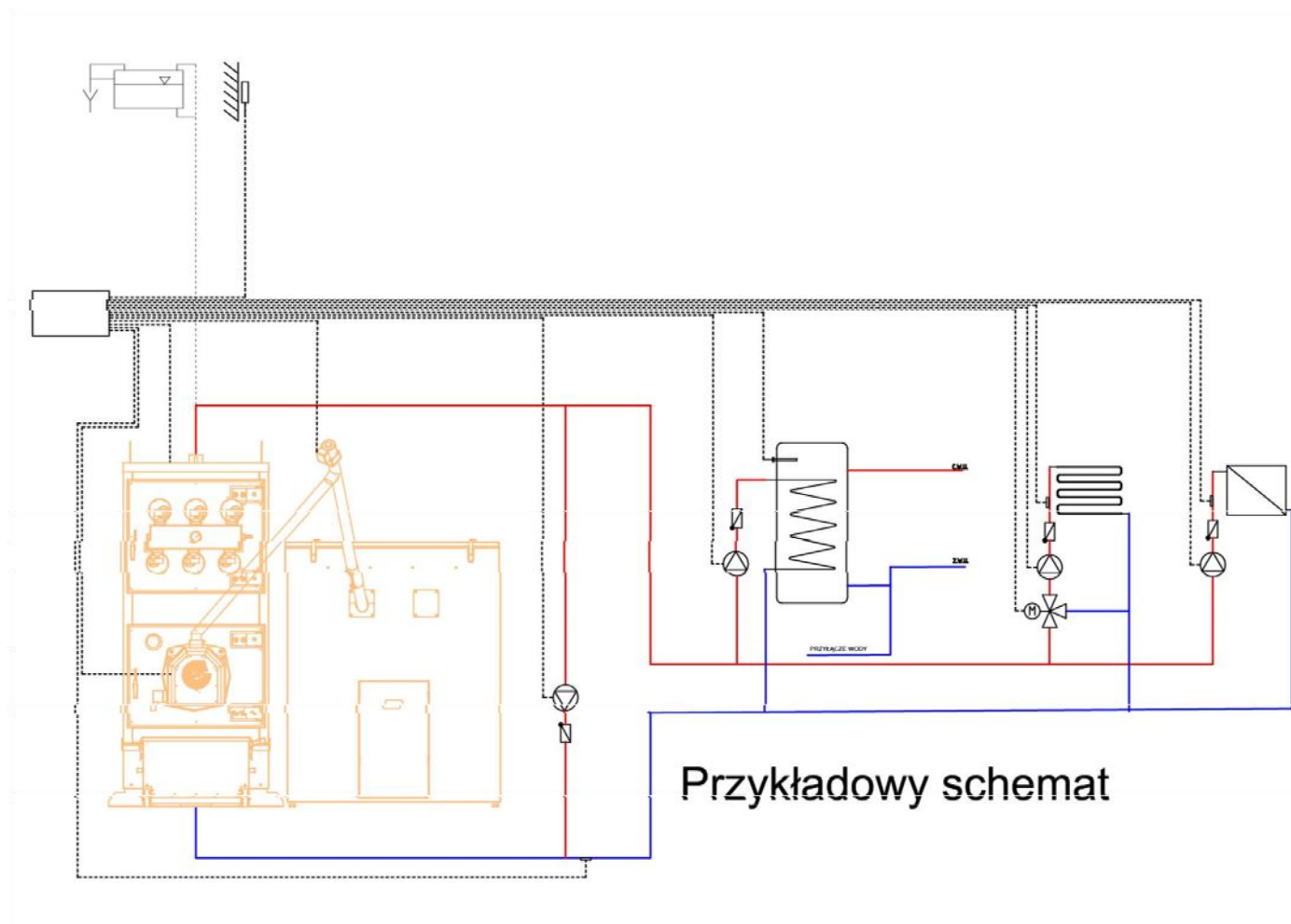
Rys. 5 Przykładowy schemat projektowanej kotłowni
