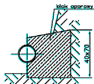
blok oporowy dla łuku
