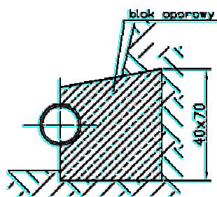
blok oporowy dla kolana
