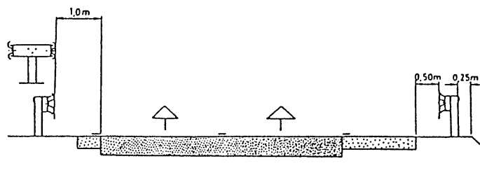
Załącznik 11.5. Dodatkowe urządzenia zabezpieczające użytkowników pojazdów jednośladowych na łukach drogi, wg [32]
