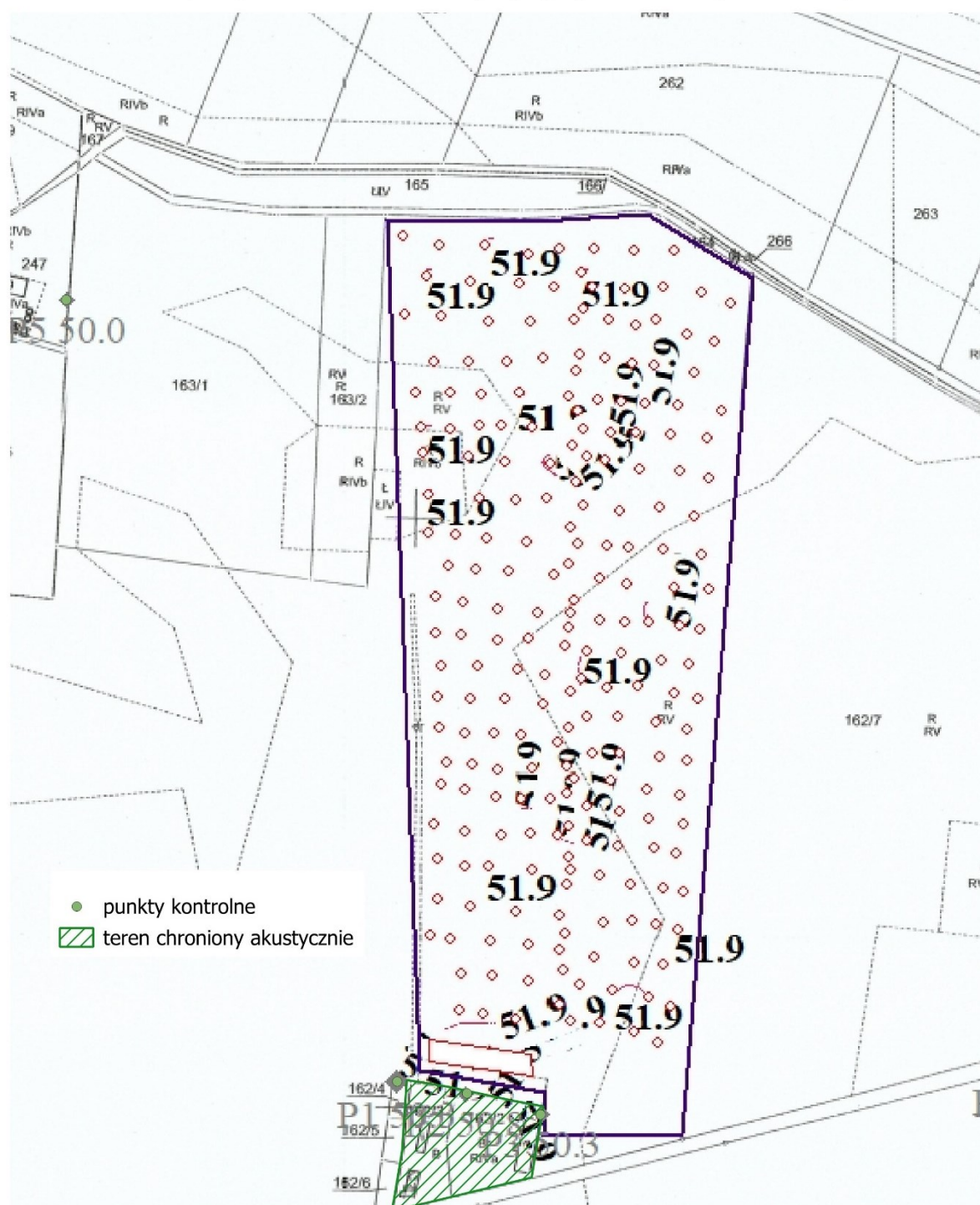
Rysunek 21 Wizualizacja wyników modelowania propagacji hałasu wariant W1b pora dnia
