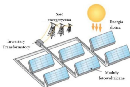
Rysunek 7 Uproszczony proces działania elektrowni fotowoltaicznej (źródło Photonlab Systemy Fotowoltaiczne AIP Jakub Wiśniewski, Politechnika Warszawska)
