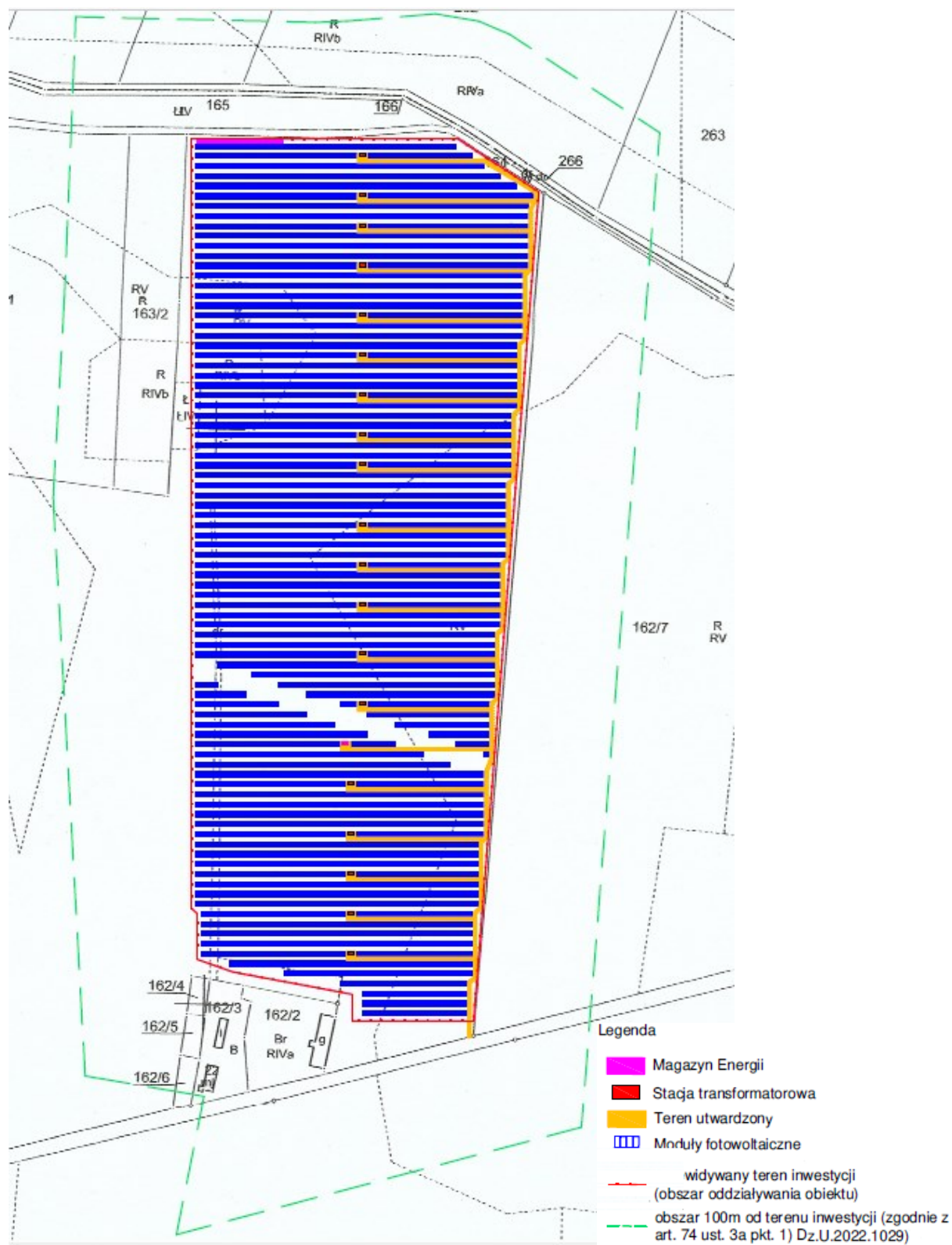
Rysunek 1 Plan zagospodarowania terenu inwestycyjnego z zaznaczonym obszarem 100 m od inwestycji.
