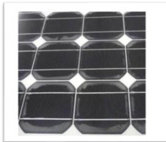
Rysunek 47 Przykład delaminacji paneli PV. Źródło: IEA International Energy Agency, Review of Failures of Photovoltaic Modules - Report IEA-PVPS T13-01:2014
