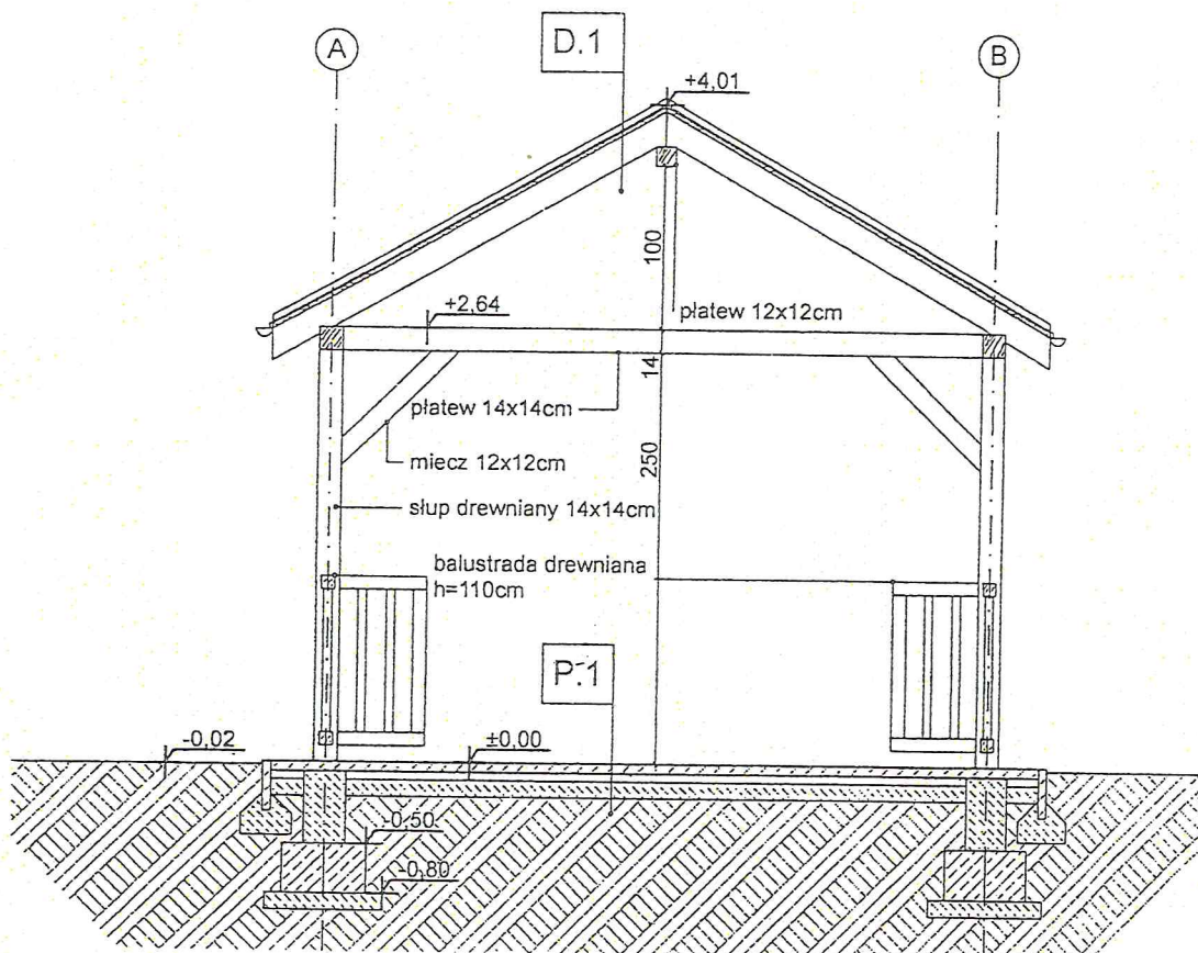
Przekrój A-A
