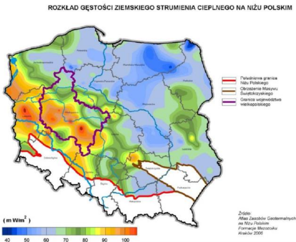
RYСУNEK 7. MAPA GĘSTOŚCI ZIEMSKIEGO STRUMIENIA CIEPLNEGO DLA OBSZARU POLSKI.
