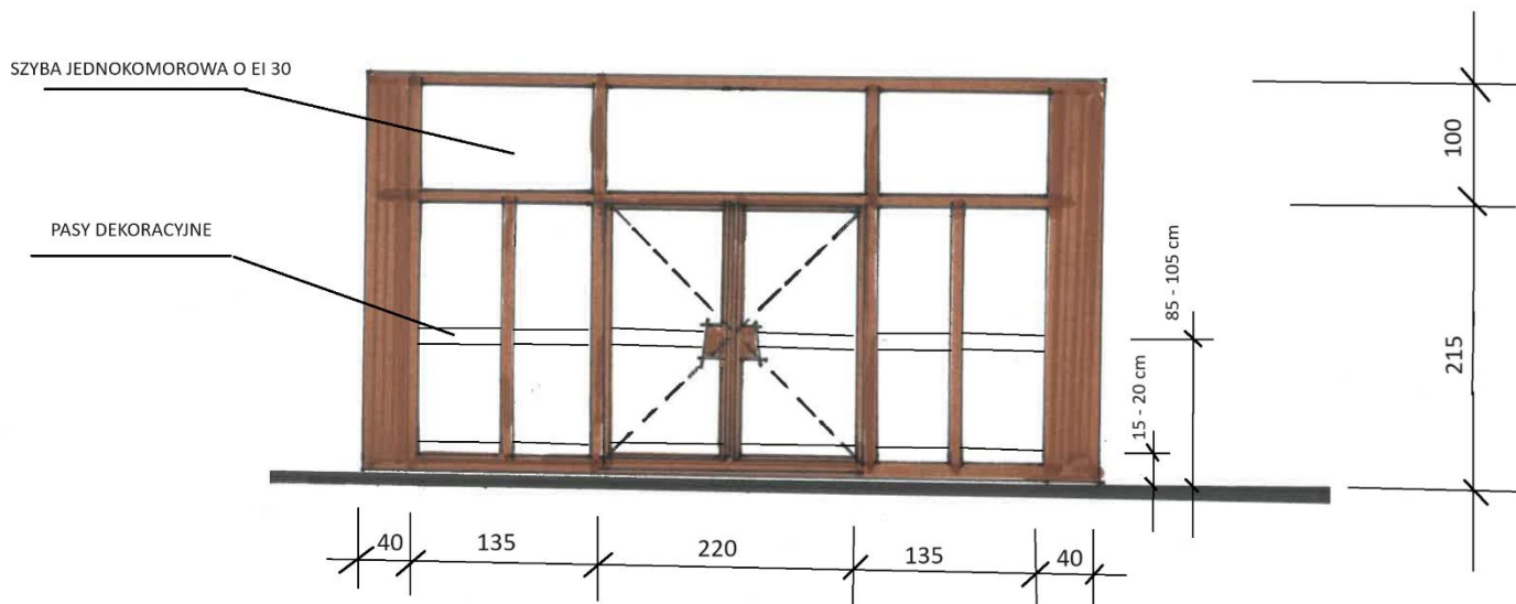
SCHEMAT ŚCIANKI PRZESZKLONEJ Z DRZWIAMI O ODPORNOŚCI OGNIOWEJ EI 30
