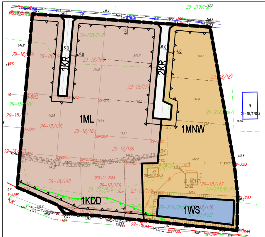
Rys. 1.6. Projekt planu.
