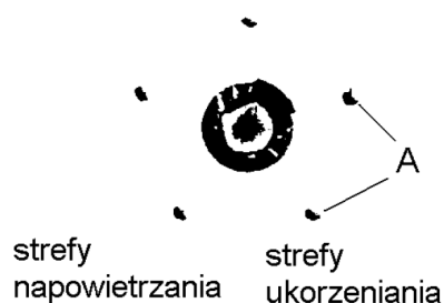
Rys. 5. Studzienka zabezpieczająca pień drzewa przy podwyższeniu terenu powyżej 0,5 m
