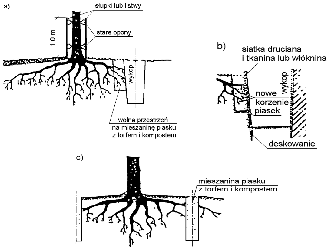
Rys. 2. Zabezpieczenie drzew przy obniżeniu terenu, po wykonaniu wykopów
