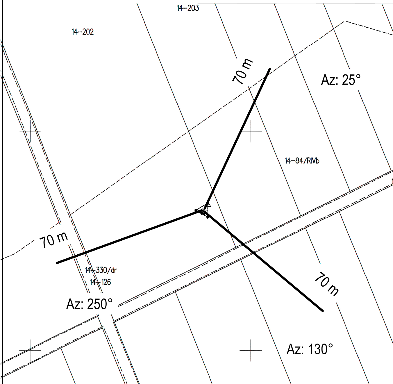
Rys. 1. Rzut poziomy osi głównej wiązki promieniowania w odległości do 40 i 70 metrów od środka elektrycznego anten sektorowych.
