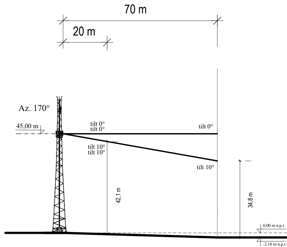
Rys. 3. Rzut pionowy osi głównej wiązki promieniowania na azymucie 170^\circ w odległości do 20 i 70 metrów od środka elektrycznego anteny sektorowej dla tiltów 0 oraz 10^\circ .
