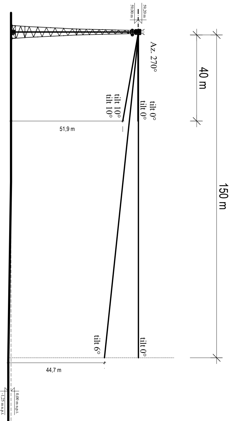
Rys. 4. Rzut pionowy osi głównej wiązki promieniowania na azymucie 270° w odległości do 40 i 150 metrów od środka elektrycznego anteny sektorowej dla tiltów 0°, 6° oraz 10°.
