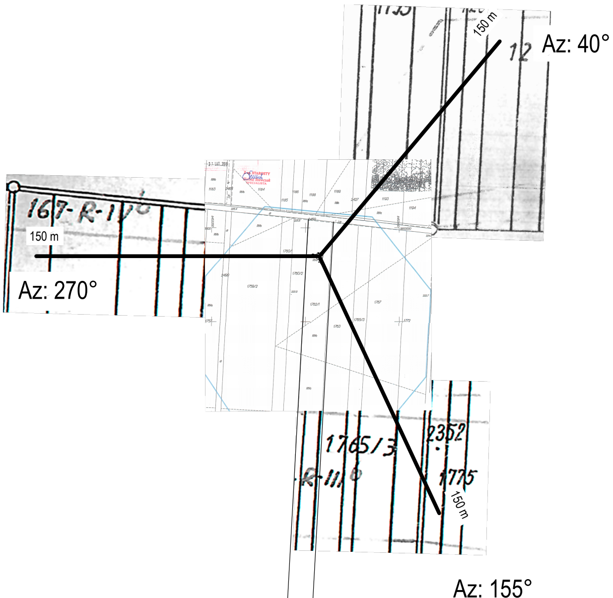
Rys. 1. Rzut poziomy osi głównej wiązki promieniowania w odległości do 40 i 150 metrów od środka elektrycznego anten sektorowych.
