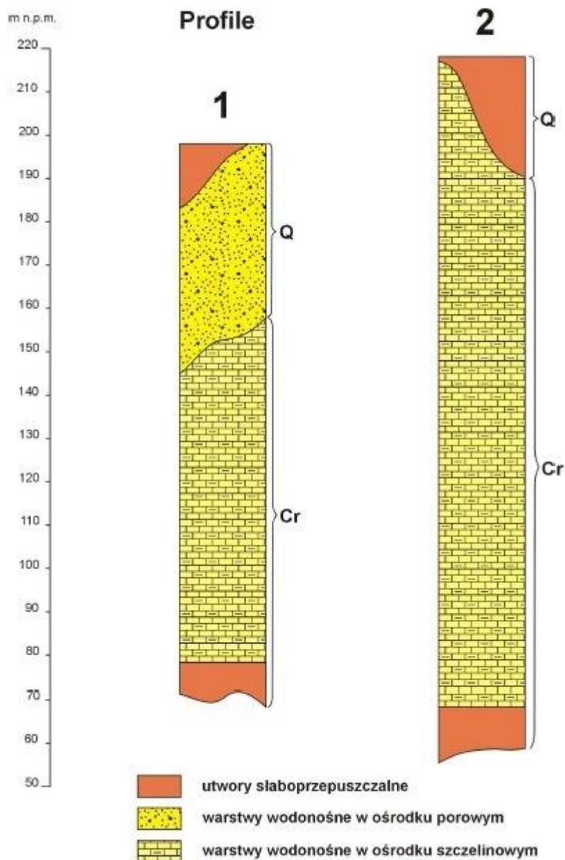
Rysunek 3.11. Profile litologiczne JCWPd 107
